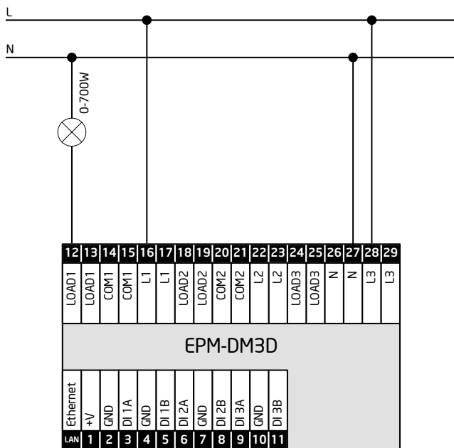
Схема 9. Использование одного канала 1.
