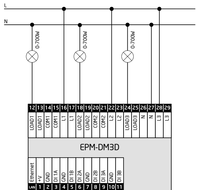
Схема 2. Три независимых канала. Три одноименных канала питания
