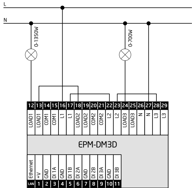
Схема 4. Объединение каналов 1+2 и 3. Один канал питания
