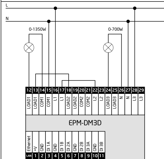
Схема 17. Объединение каналов 1+2 и 3. Использование контактов COM1 и N для подключения нейтрали от нагрузки
