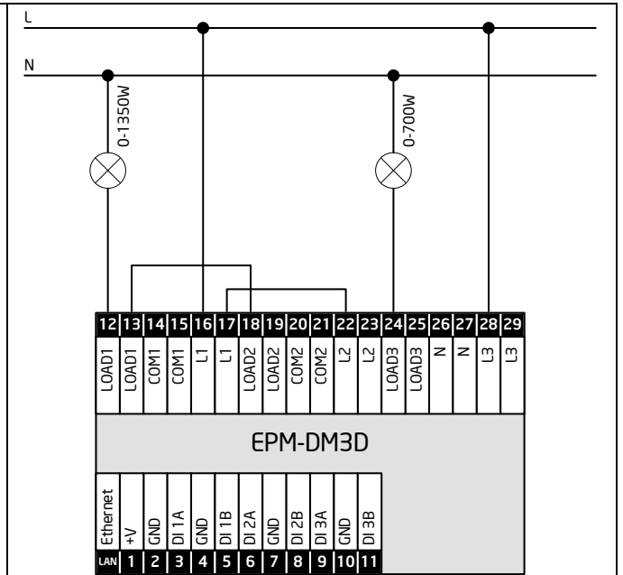
Схема 16. Объединение каналов 1+2 и 3. Две одноименных фазы по каждому каналу питания
