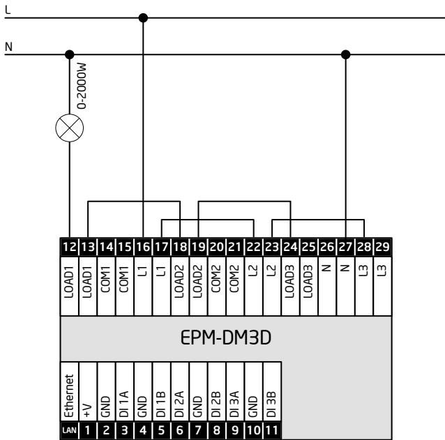
Схема 7. Объединение каналов 1+2+3. Один канал питания
