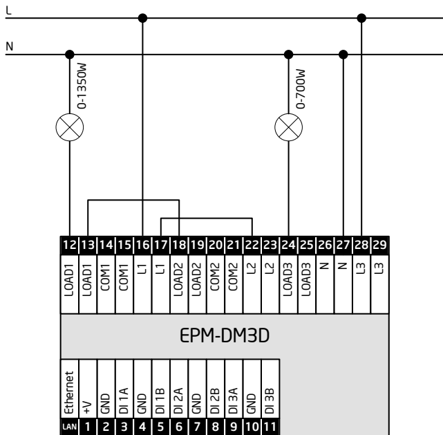
Схема 5. Объединение каналов 1+2 и 3. Два одноименных канала питания
