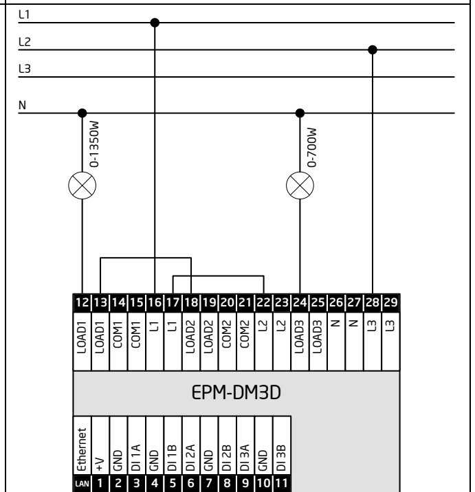
Схема 18. Объединение каналов 1+2 и 3. Две разноименных фазы по каждому каналу питания
