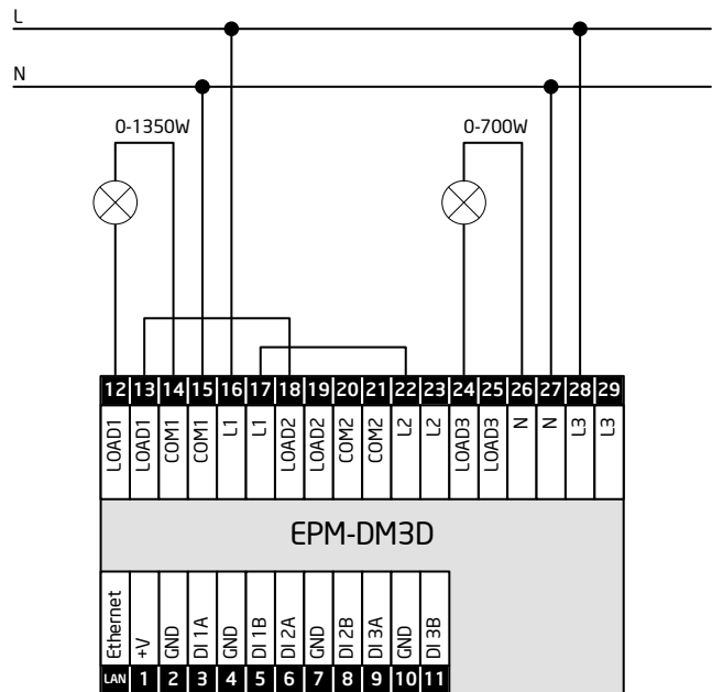
Схема 6. Объединение каналов 1+2 и 3. Два одноименных канала питания. Использование контактов COM1 и N для подключения нейтрали от нагрузки
