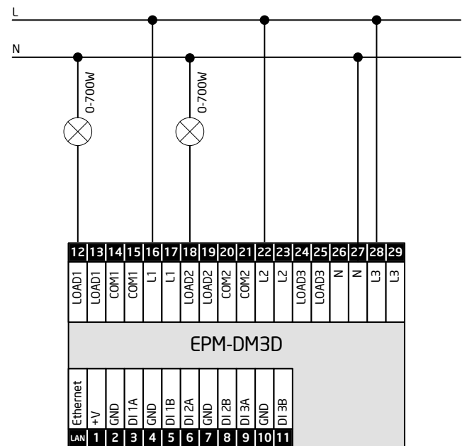
Схема 10. Использование двух каналов 1 и 2.
