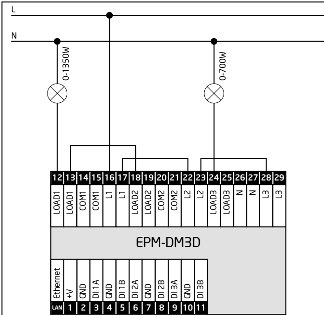
Схема 15. Объединение каналов 1+2 и 3. Один канал питания
