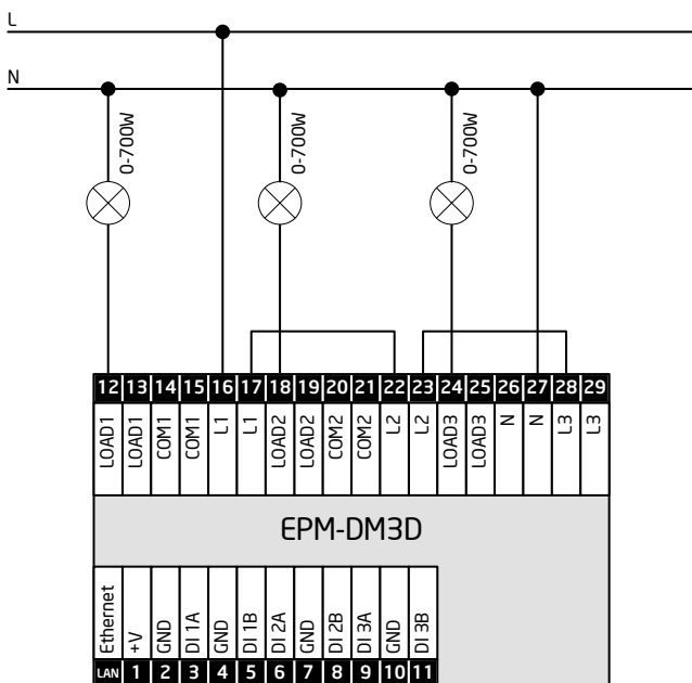
Схема 1. Три независимых канала. Один канал питания
