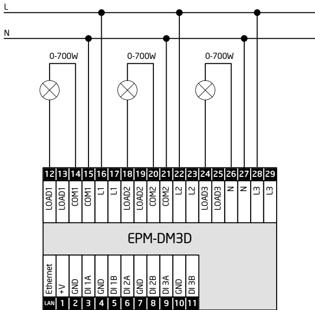
Схема 3. Три независимых канала. Использование контактов COM1, COM2 и N для подключения нейтрали от нагрузки
