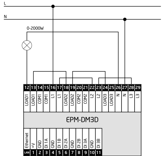
Схема 8. Объединение каналов 1+2+3. Один канал питания. Использование контактов N для подключения нейтрали от нагрузки
